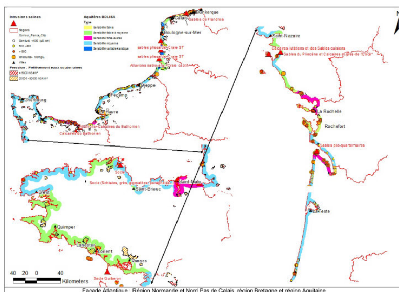
Carte de vulnérabilité des nappes souterraines vis-à-vis d'une intrusion saline pour une bande littorale de 5 km de large.
