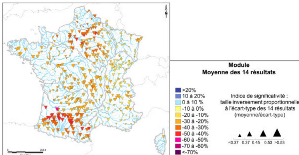
Figure 1 : Evolutions relatives possibles (en %) du débit moyen annuel entre 1961-90 et 2046-65 : Résultats moyens établis sur les 14 simulations (2 modèles hydrologiques x 7 MCG). La couleur des points est fonction de l'intensité du changement et la taille des points est liée à la convergence des 14 simulations.
