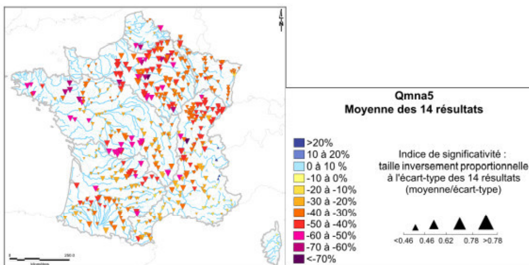
Figure 3 : Evolutions relatives possibles (en %) du QMNA5 entre 1961-90 et 2046-65 : Résultats moyens établis sur les 14 simulations (2 modèles hydrologiques x 7 MCG).
